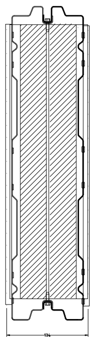
1:2 Przekrój
