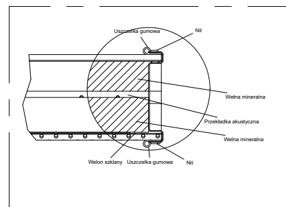
1:20 Szczegół J
